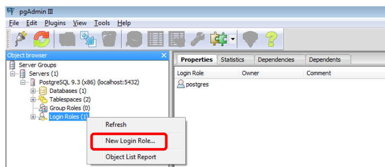
FIGURA 74. Creación del rol admbonitabpm para la base de datos GestionDocumental
