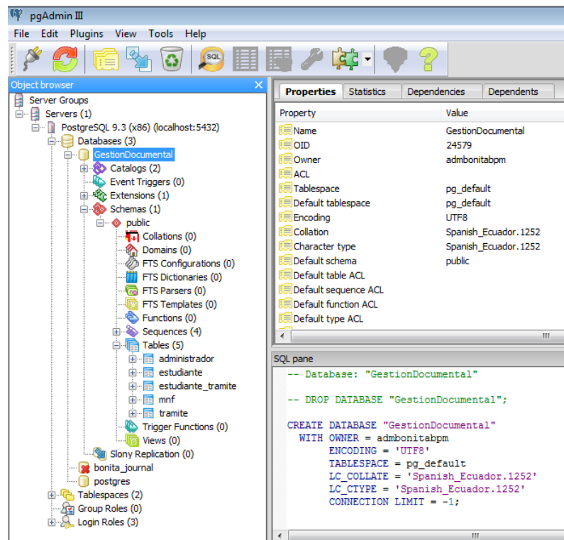
FIGURA 84. Esquema de la Base de datos GestiónDocumental
