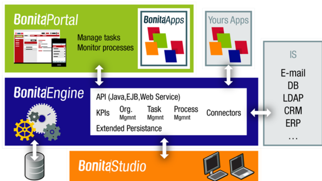
FIGURA 1. Componentes de BonitaSoft
