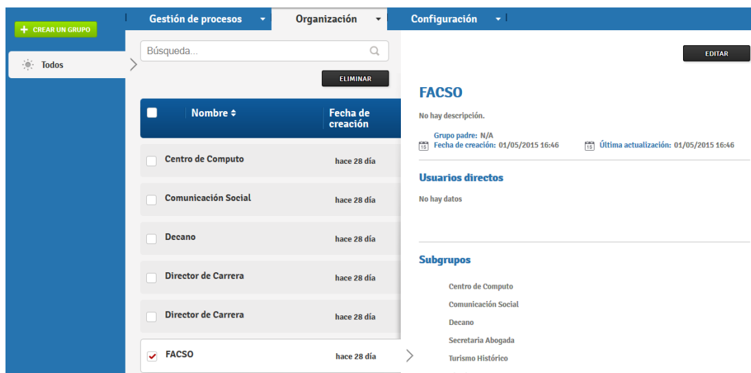
FIGURA 156. Subnivel Grupos
