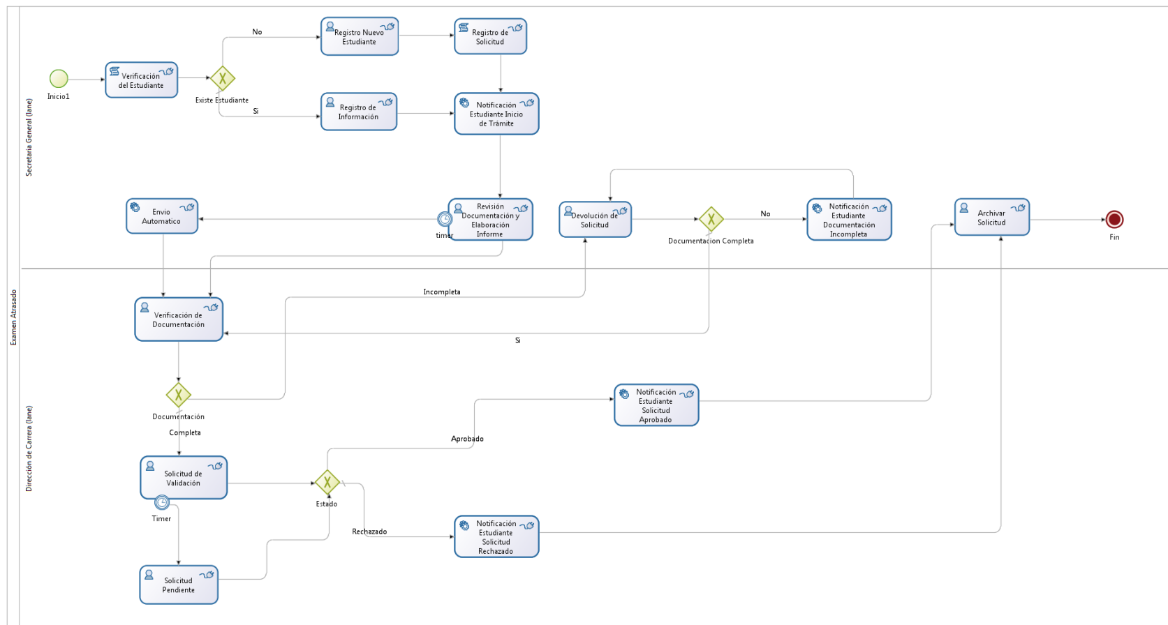
FIGURA 25. Diagrama Recalificación
