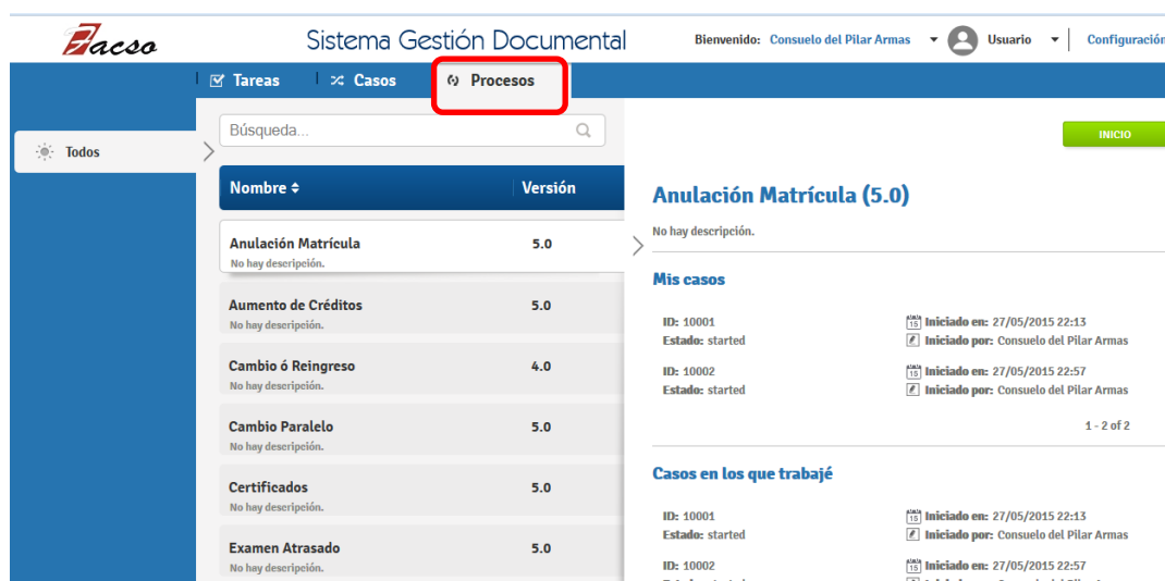
FIGURA 170. Procesos
