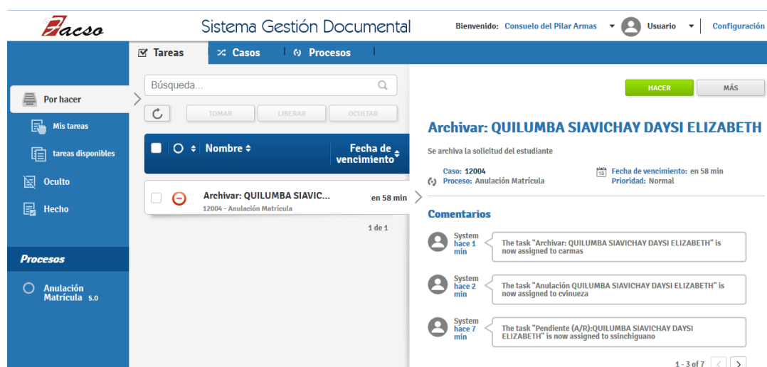
FIGURA 184. Tarea Archivar
