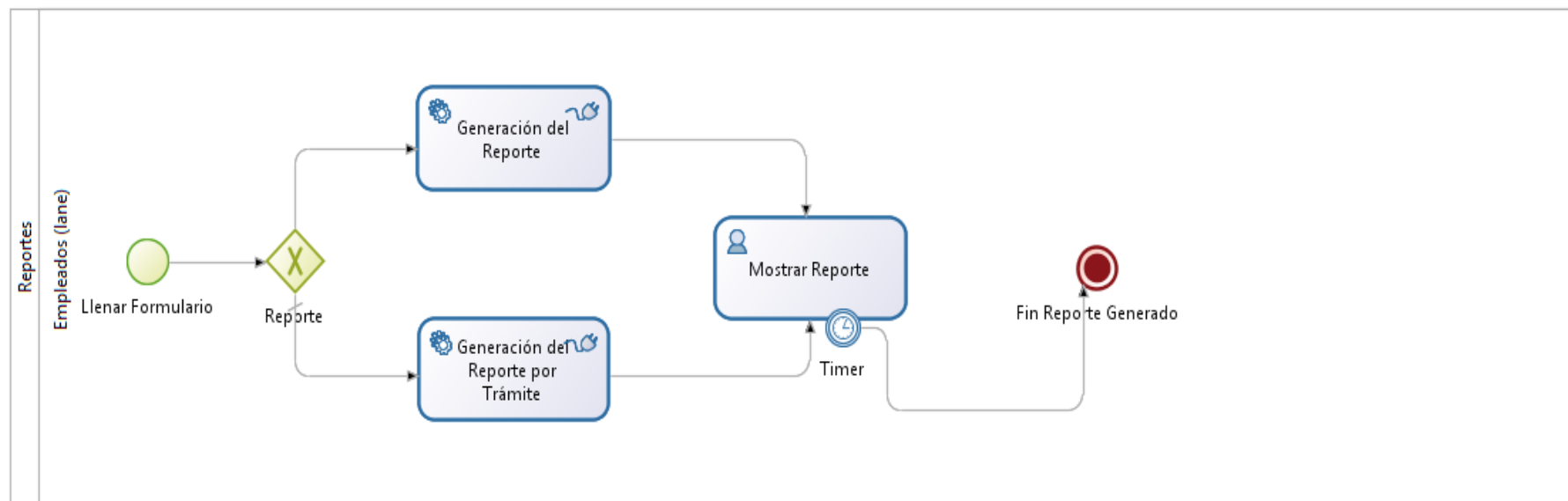
FIGURA 30. Diagrama Reportes
