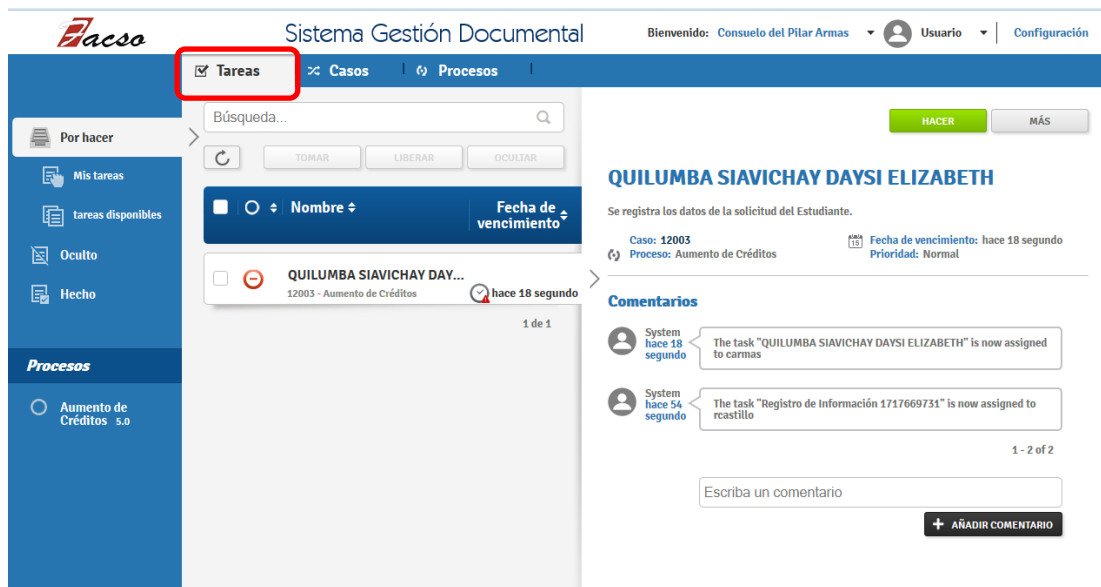
FIGURA 168. Tareas
