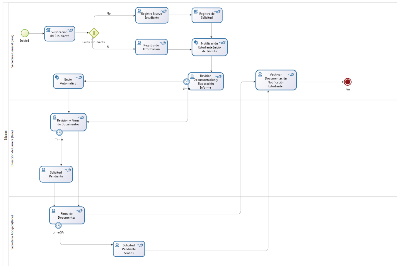
FIGURA 22. Diagrama Sílabos
