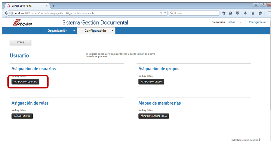
FIGURA 123. Privilegios Usuario
