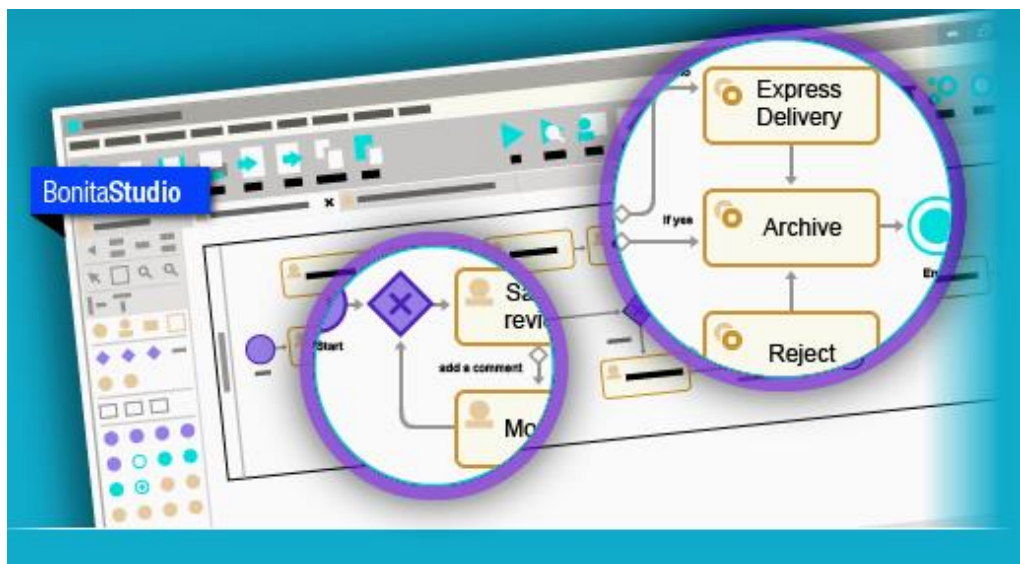
FIGURA 19. Bonita Studio
