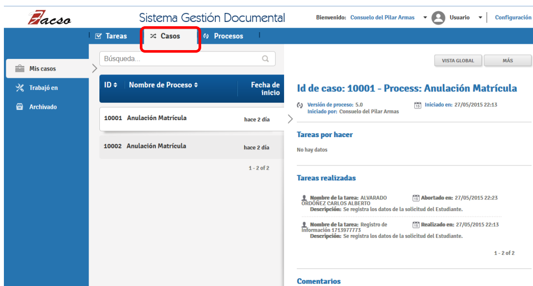
FIGURA 169. Casos
