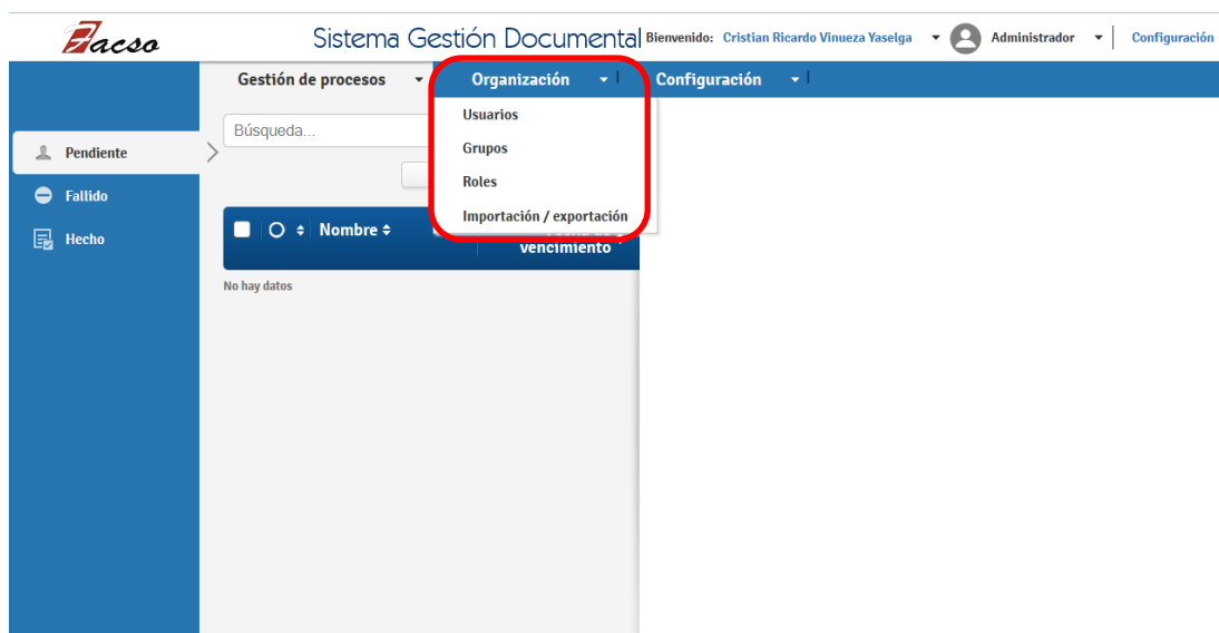
FIGURA 151. Nivel Organización
