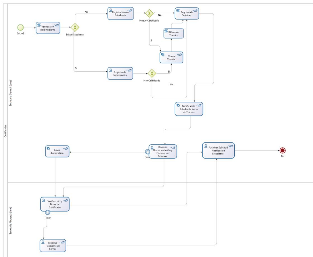
FIGURA 29. Diagrama Certificados
