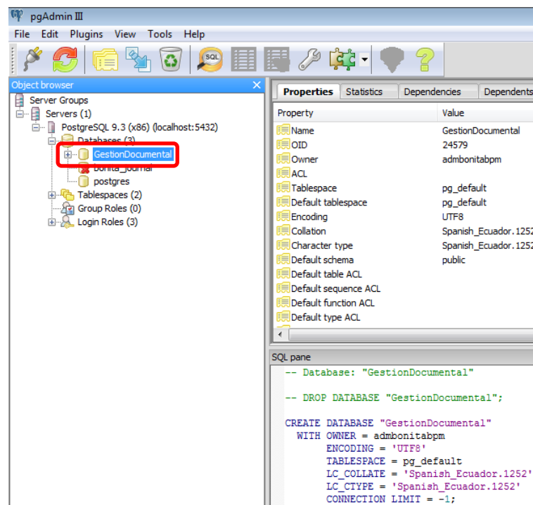
FIGURA 80. Base de Datos GestionDocumental
