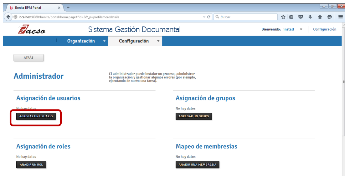
FIGURA 118. Privilegios Administrador (2)
