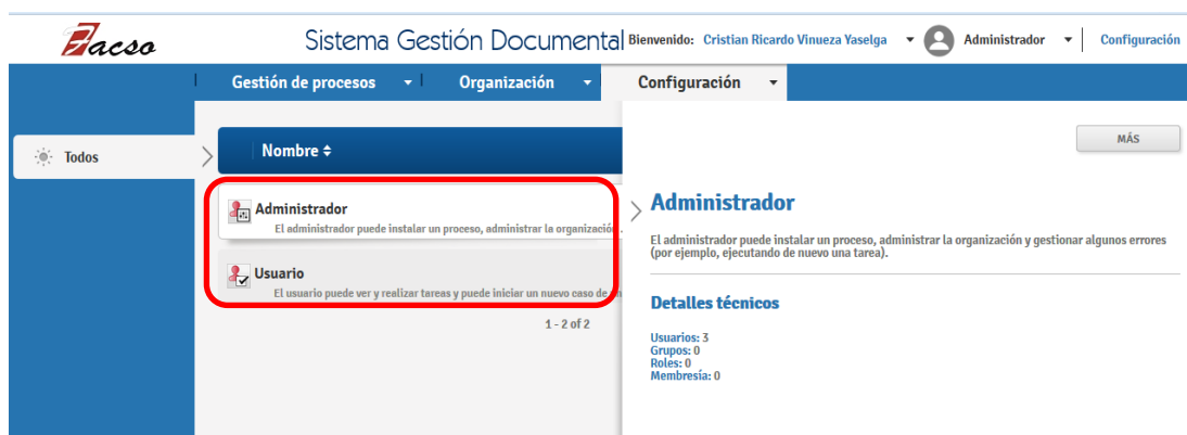
FIGURA 164. Subnivel Privilegios
