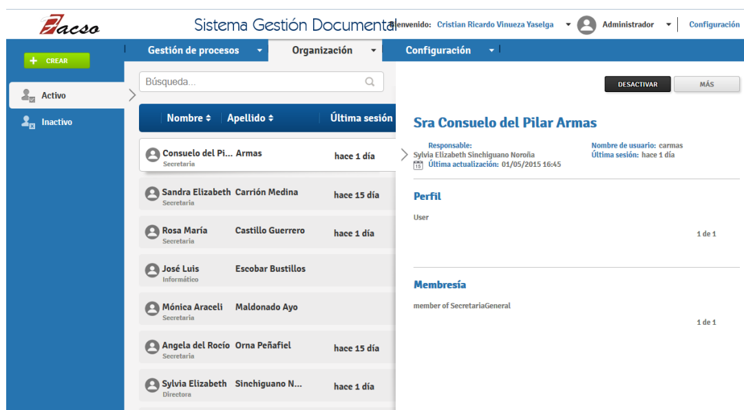
FIGURA 152. Subnivel Usuarios
