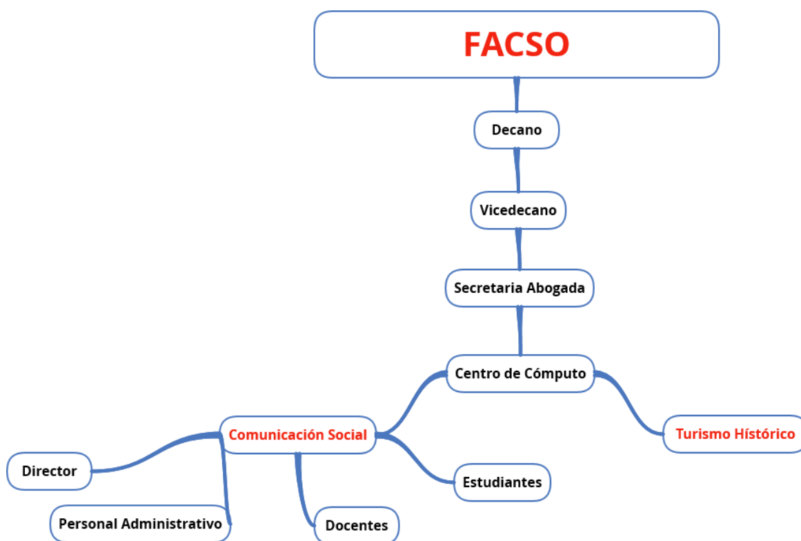
FIGURA 150. Organización FACSO
