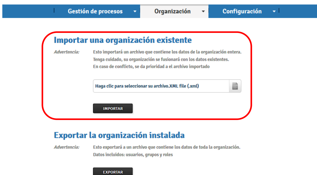
FIGURA 161. Subnivel Importación/exportación
