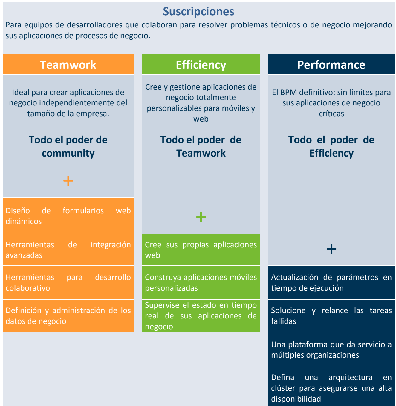
FIGURA 9. Edición Suscripción
