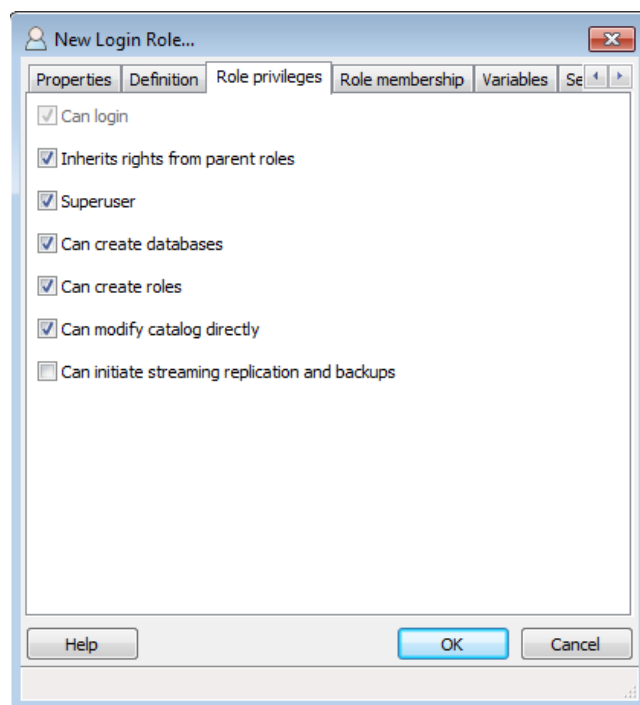
FIGURA 70. Selección de los privilegios para el rol bonita
